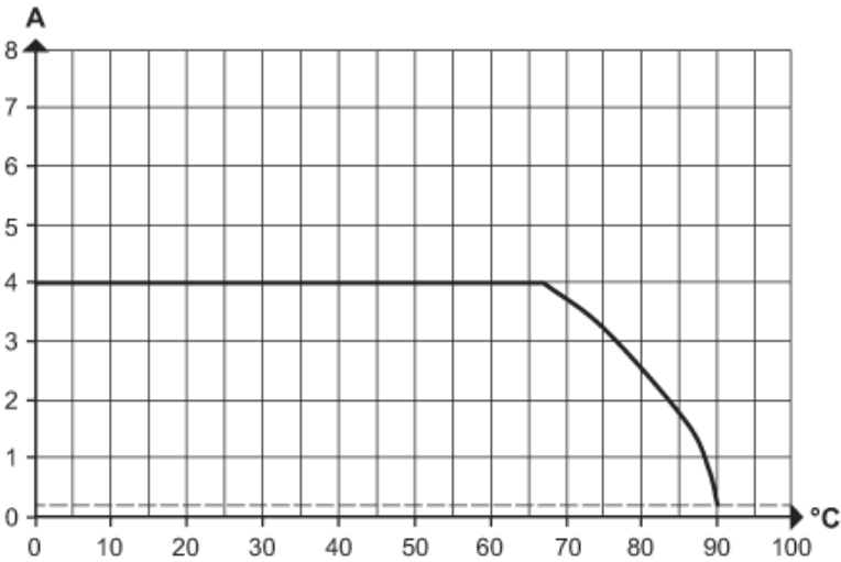
Снижение мощности I_{max} * 0.8 (DIN EN 60512-5-2)
